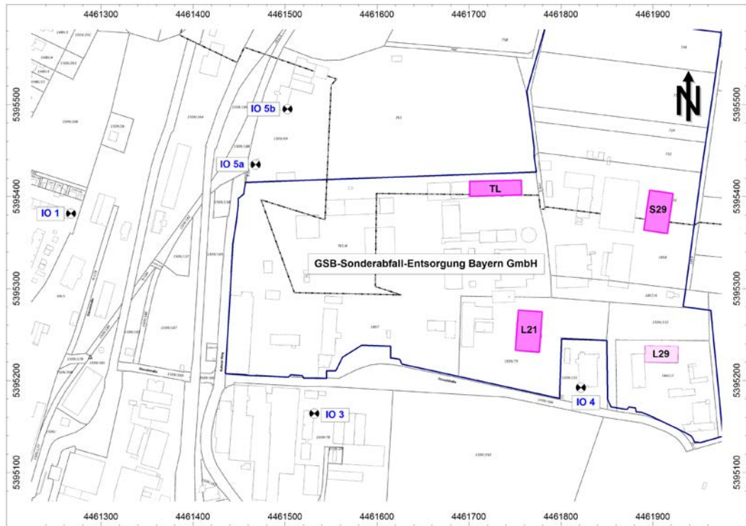
Abbildung 1. Lageplan der Bautätigkeiten und der Immissionsorte.
